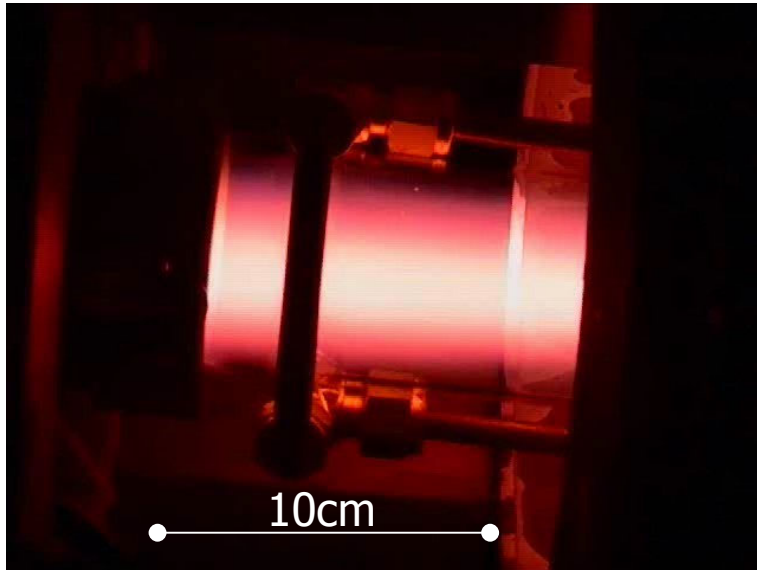
Helium
